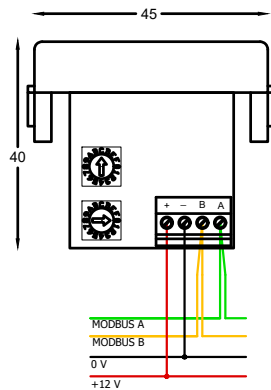
Conexión al Sistema Modbus
