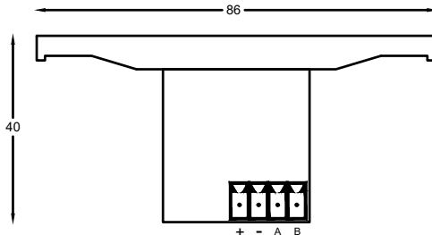
Conexión al sistema Modbus
