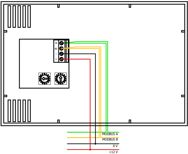
Vista posterior (sin placca de cubierta)
