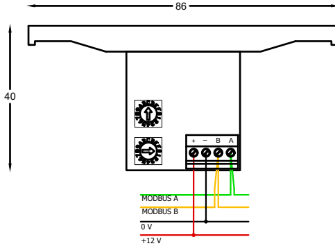
Conexión al sistema Modbus
