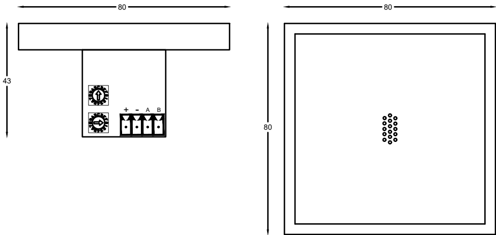
Elemento con microprocesador y sensor
